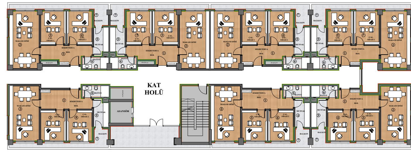
A BLOK 1. GİRİŞ 1. KAT PLANI
